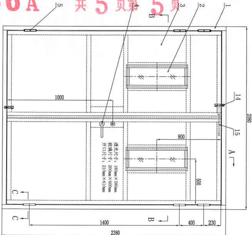
背火面立面图
