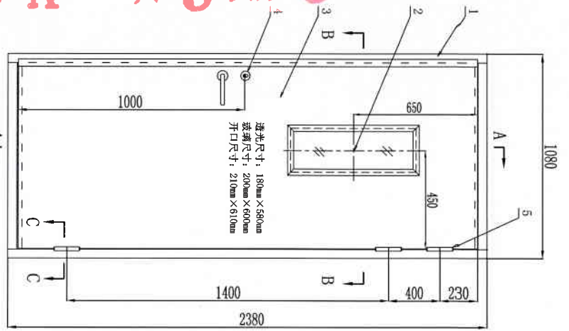
背面立面图
